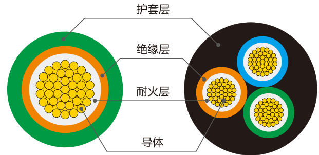
N-BVV结构示意图 ( 10mm²及以上 )
