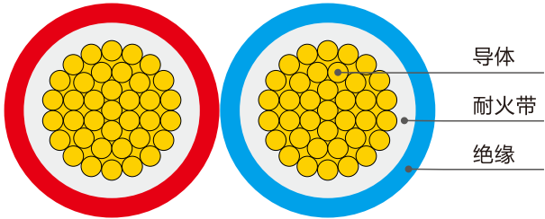
WDZN-RYS、WDZN-RYJS结构示意图
