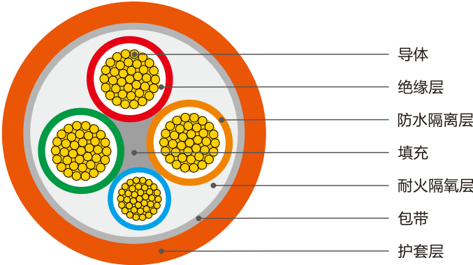
BBTRZ结构示意图
