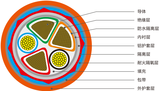
BTLY结构示意图
