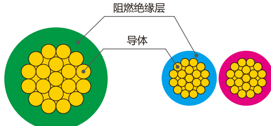
Z(A,B,C)-BVR及BVR结构示意图
