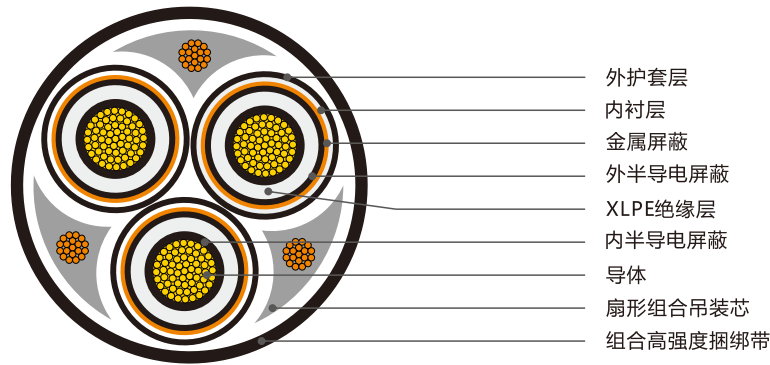
DZ-WDZA-YJY、DZ-WDZB1-YJY结构示意图
