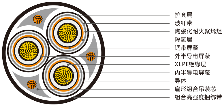
DZ-WDZAN-YJY、DZ-WDZB1N-YJY结构示意图
