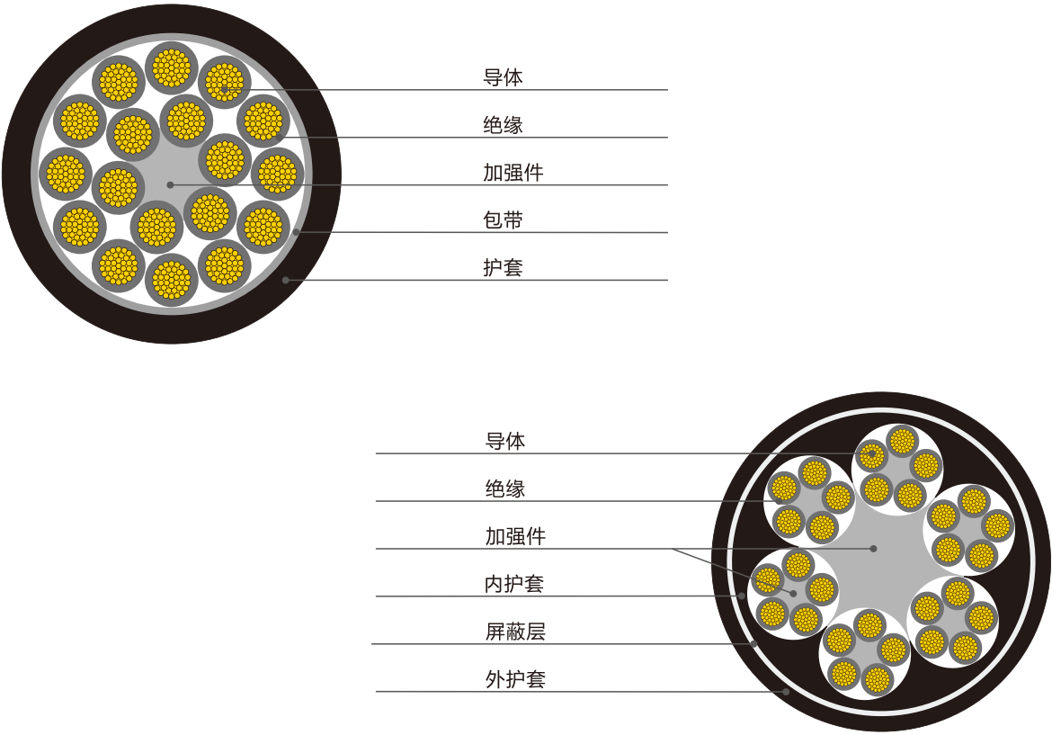
拖链控制电缆结构示意图
