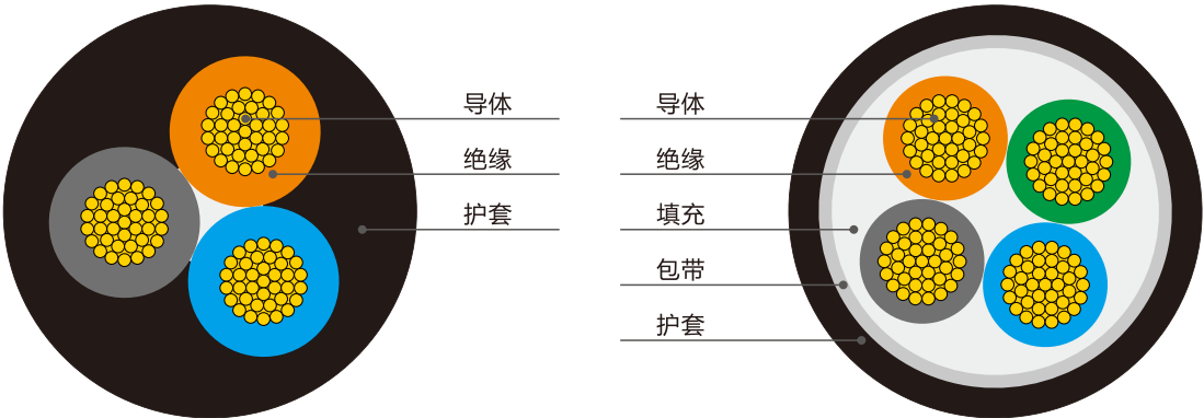
多芯屏蔽（可选）护套线结构示意图
