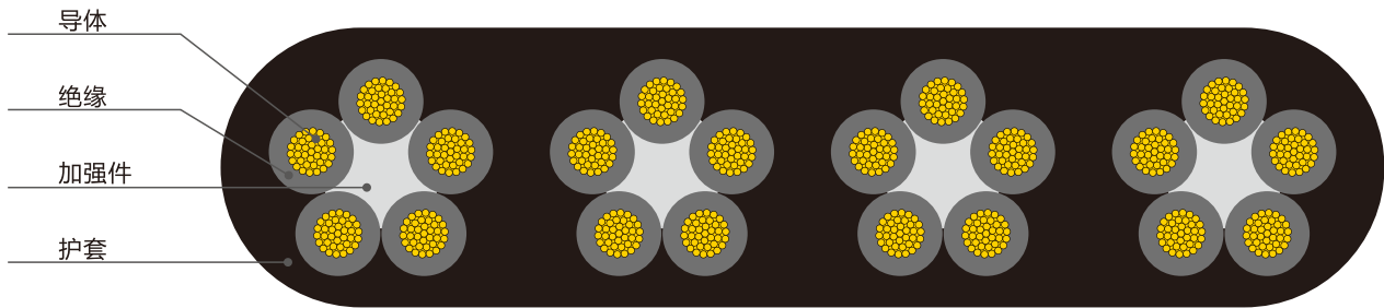
TVVB结构示意图
