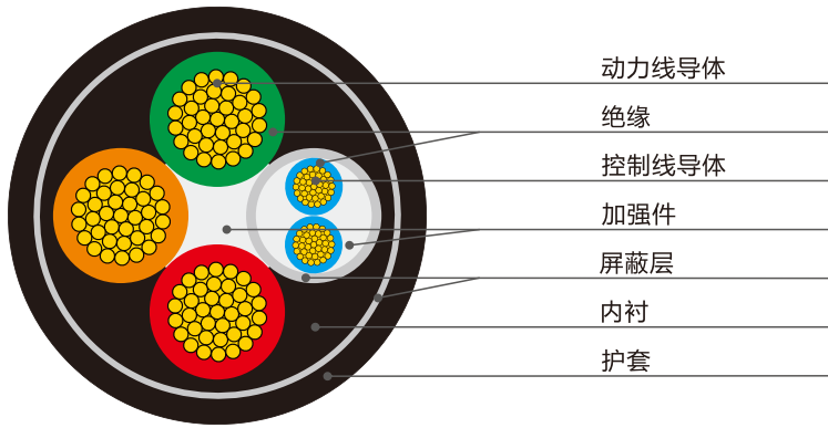
拖链伺服电缆结构示意图
