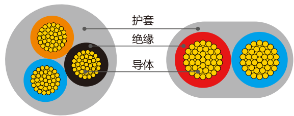
RVV结构示意图
