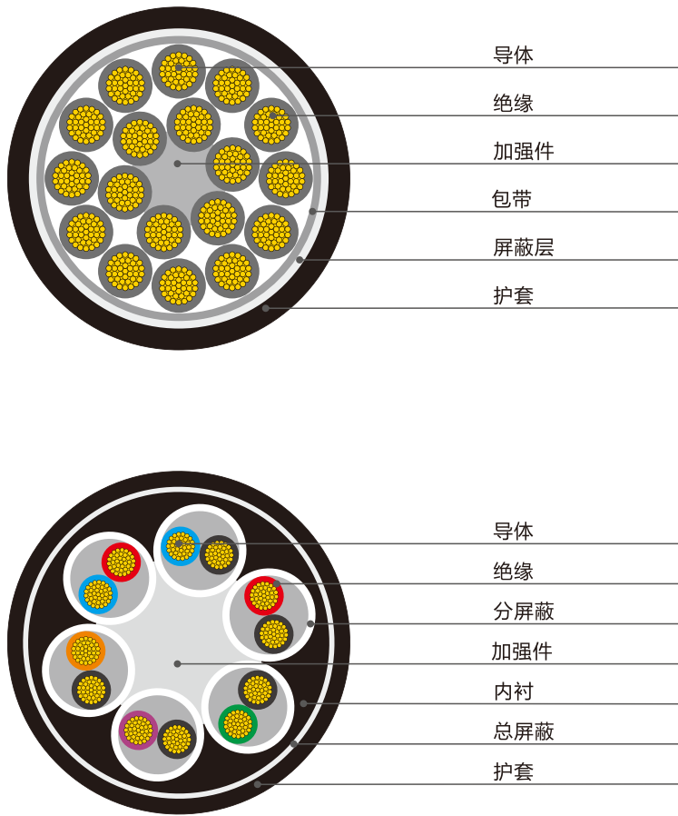
拖链数据电缆结构示意图
