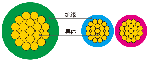
AVR、BV、RV、BVR结构示意图 RVS结构示意图
