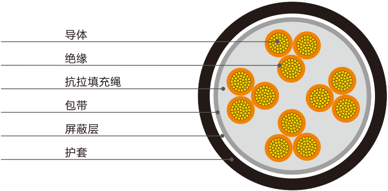
行车控制电缆结构示意图
